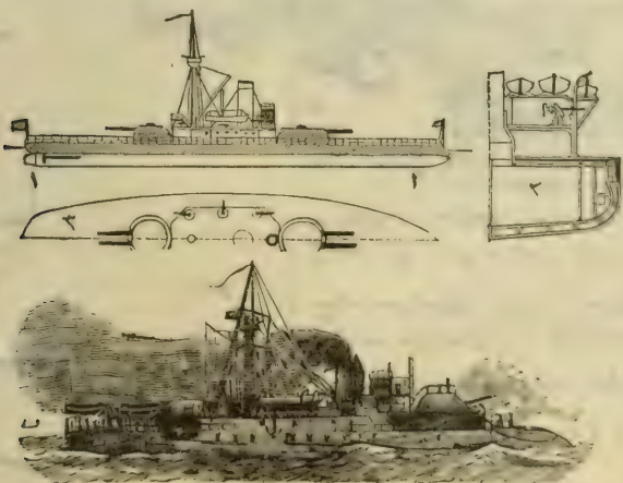
( ساحل محافظه سنه مخصوص سفینه حریره )
